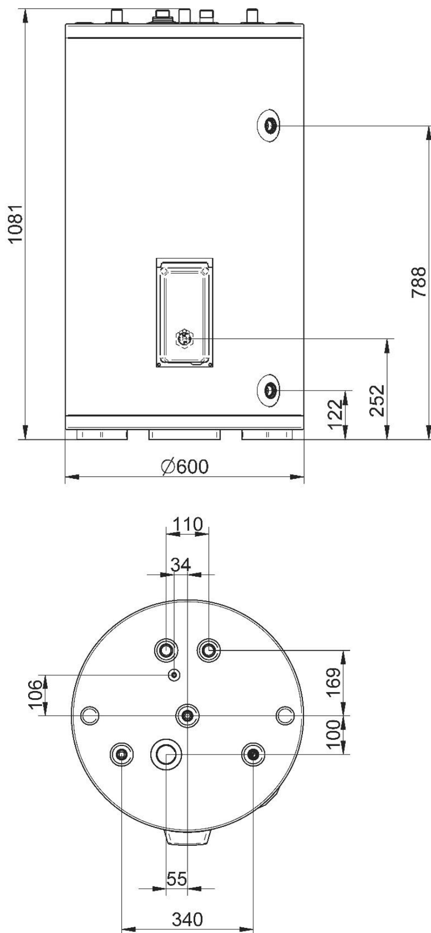
Рис. 6. Габаритные размеры водонагревателя UBC 150
